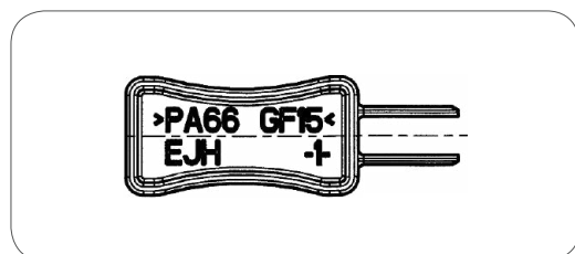
Entriegelungswerkzeug für MCP 2,8mm Kontakte Unlocking tool for MCP 2.8mm contacts
